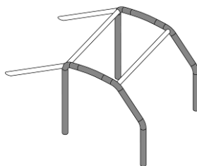
2 oldalsó bukócső / lateral rollbars 2 keresztmerevítő / transverse members 2 hátsó megtámasztás / backstays
