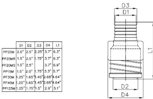
Gyorscsatlakozó sorozat csavar / Push pull series male
