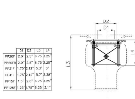
Gyorscsatlakozó sorozat anya / Push pull series female
