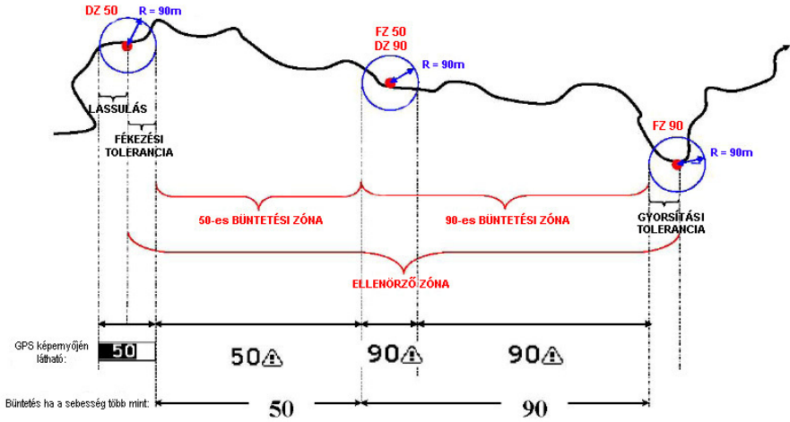
D ábra: EGYMÁS UTÁNI SEBESSÉGELLENŐRZÖTT ZÓNÁK EMELKEDŐ SEBESSÉGGEL 50-ről 90-re
