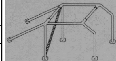
Dessin/drawing n° 253-9
