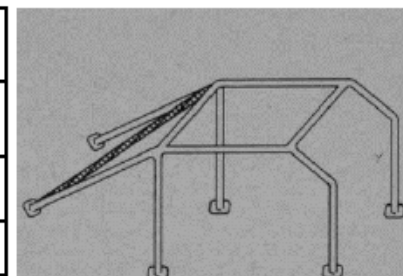
Dessin/drawing n° 253-8
