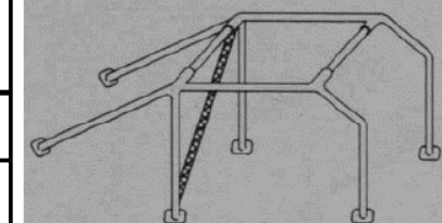
Dessin/drawing n° 253-9
