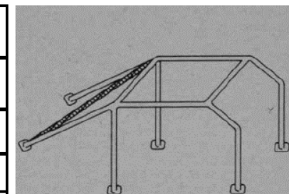
Dessin/drawing n° 253-8
